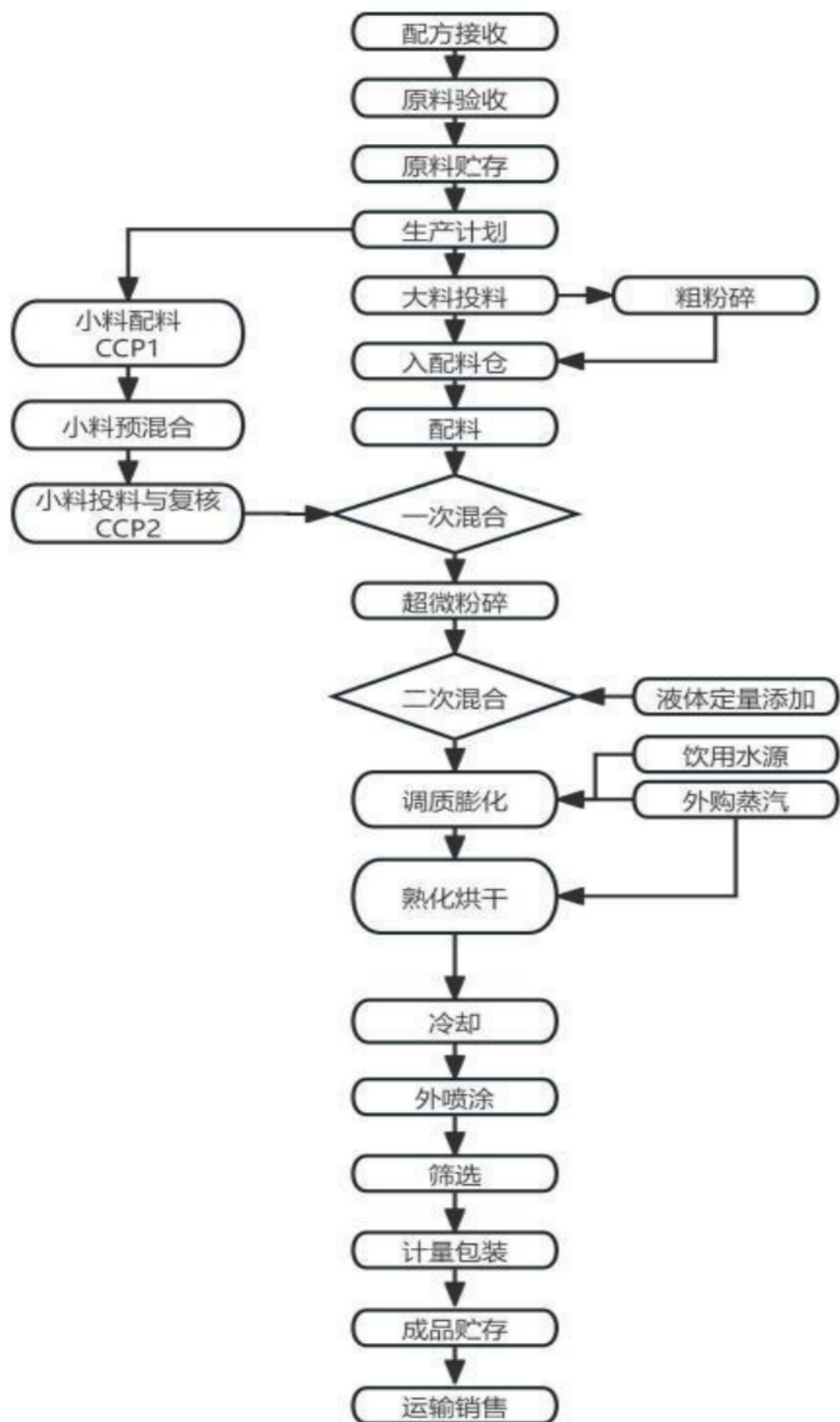
受核查方生产工艺流程图
